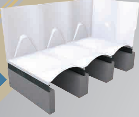
TABANI DIŞTAN FLANŞLI GRP MODÜLER SU DEPOSU
