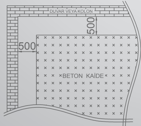
BETON KAİDE ÖN GÖRÜNÜŞÜ
